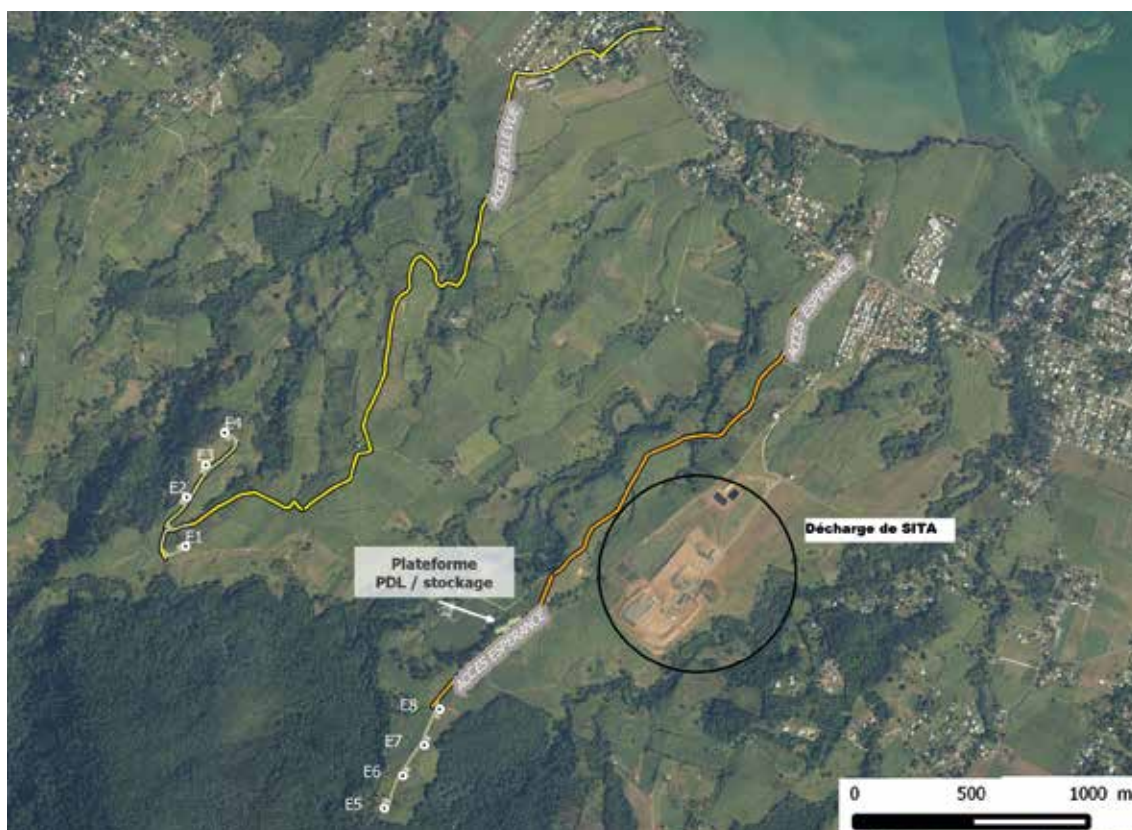
Implantation des 8 éoliennes de Sainte-Rose (E1 à E8)
